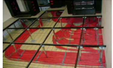
Figura 11: Cabos organizados sob piso elevado
