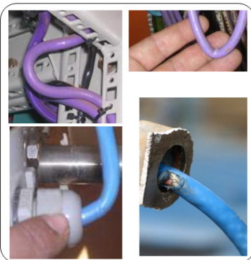
Figura 9: Exemplos de cabos NÃO respeitando o seu raio de curvatura
